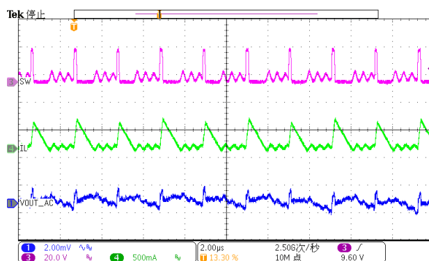
Figure 22. Output Ripple (Iload=100mA)
